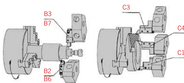
Einsatz von Werkzeughaltern bei rechter Spindeldrehrichtung Application of toolholders with clockwise spindle rotation
