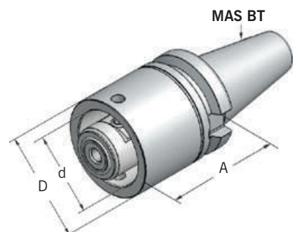
MAS BT
