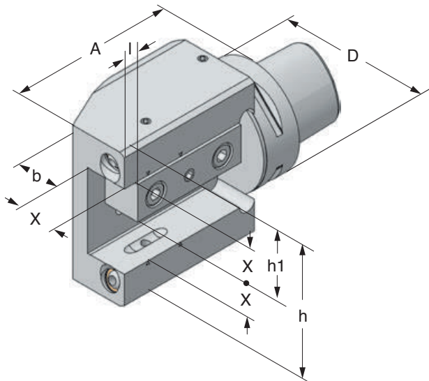
ISO 26623 - C6
