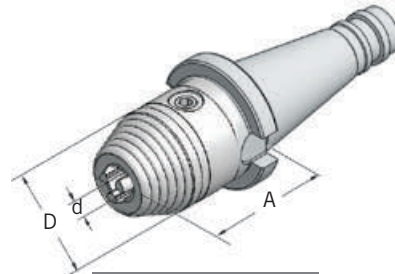
DIN 2080
