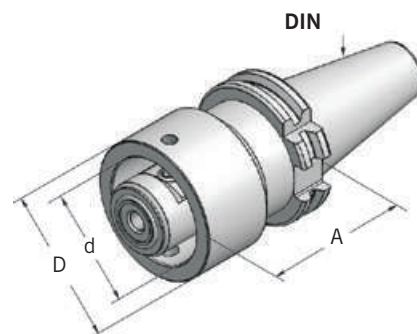
DIN 69871
